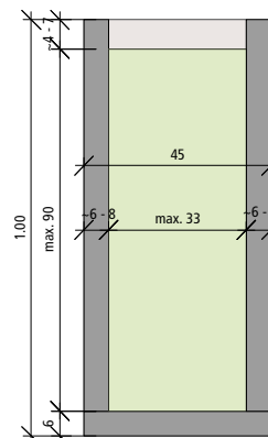
Aufsicht
