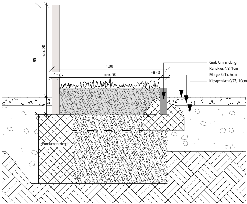
Längsschnitt
