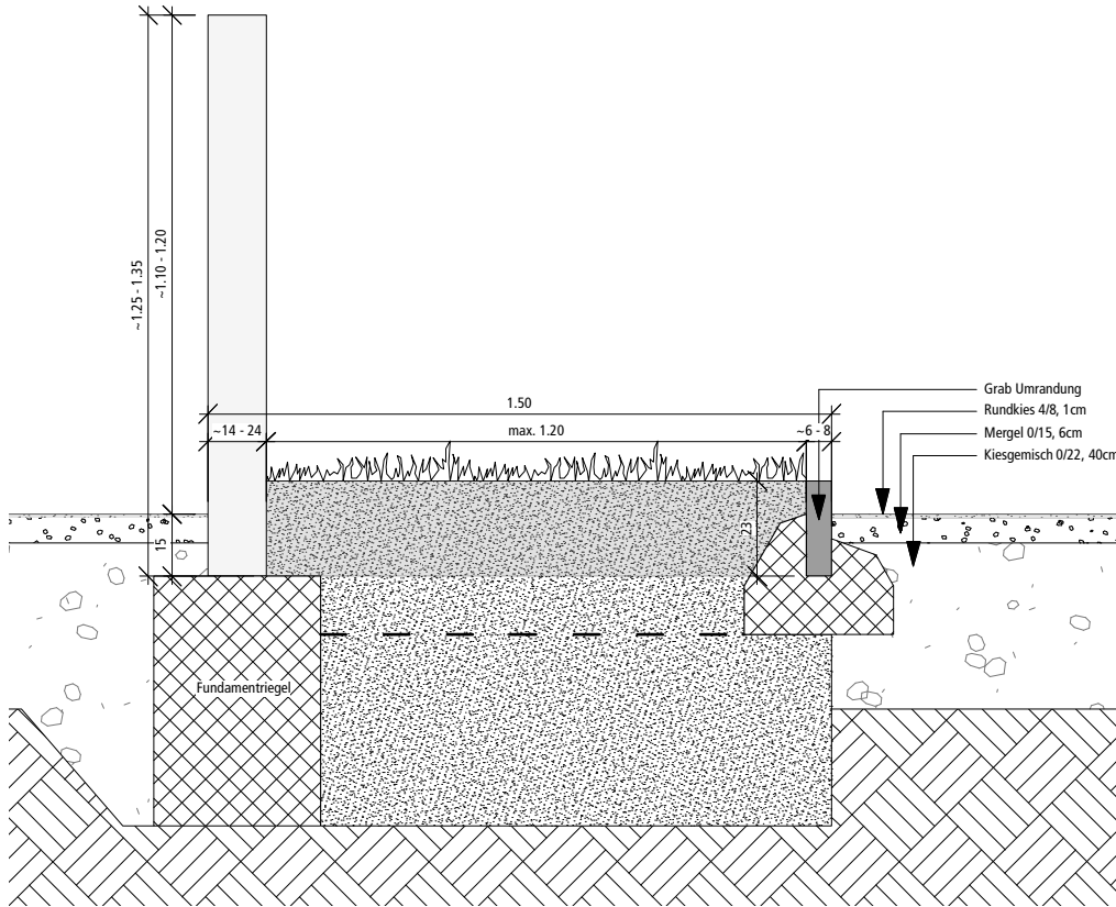
Längsschnitt
